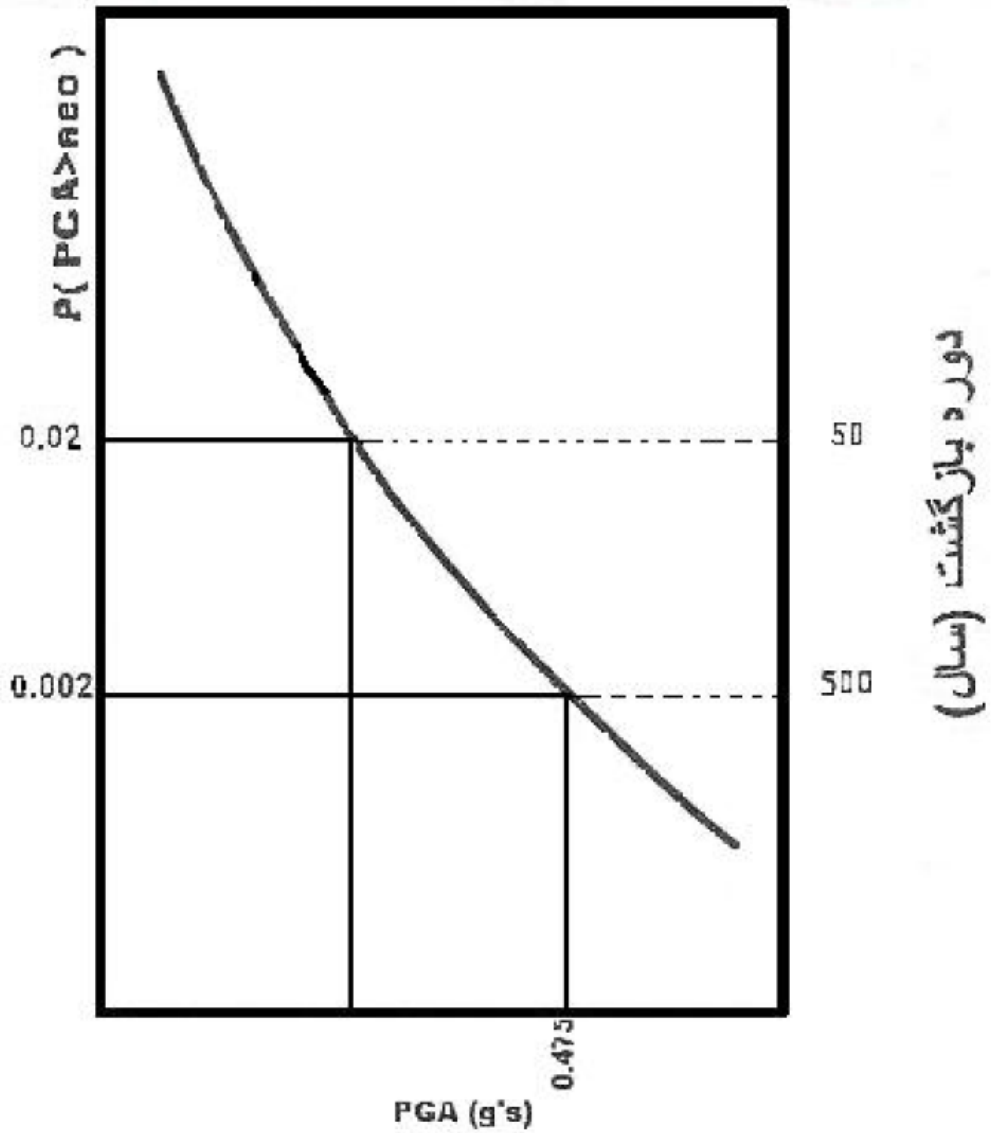
شکل (ت ۳-۱): منحنی خطر براساس احتمال وقوع (یا دوره بازگشت به سال)
